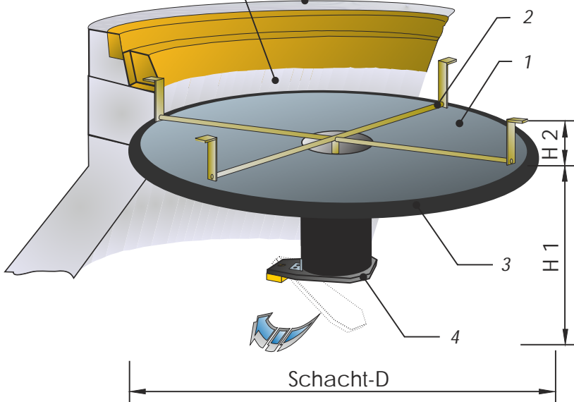
Ausgleichsring mit Schachtkonus
